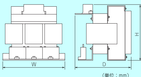
《FR-ASF》
