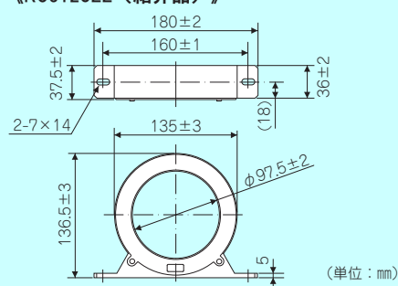
《RC5128ZZ (紹介品)》
