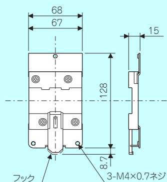
《FR-UDA01》
