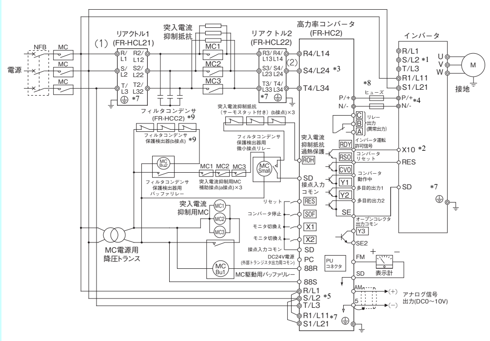
《FR-HC2-H400K、H560K》
