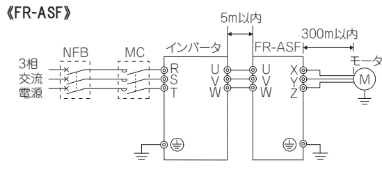
《FR-ASF》
