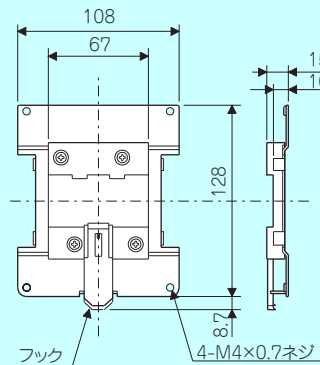
《FR-UDA02》
