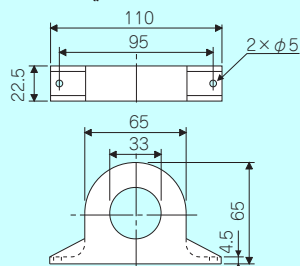
《FR-BSF01》
