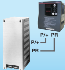
ブレーキユニット (FR-BU2)
